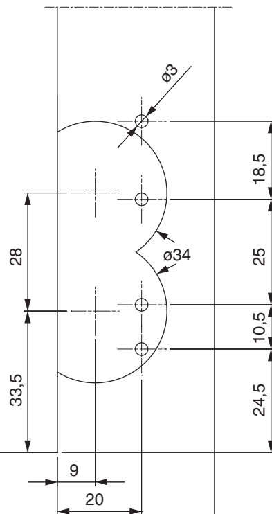
Supporto cerniera doppia tazza 12/20 per portafinestre
