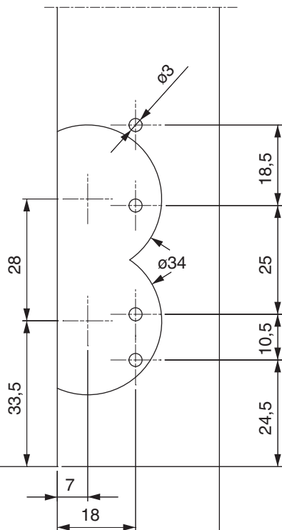
Supporto cerniera doppia tazza 12/18 per portafinestre
